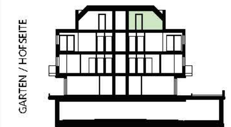
SCHNITT
